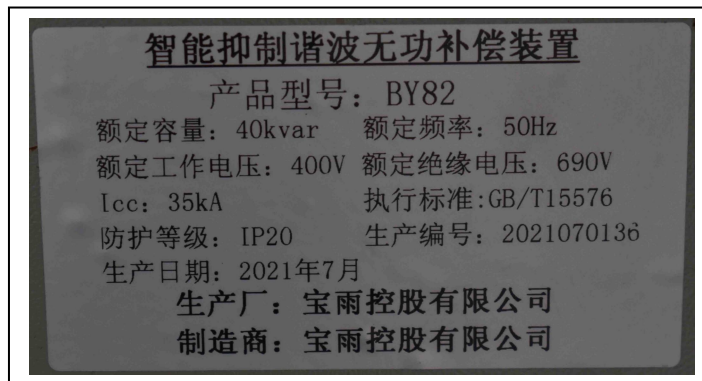
铭牌
